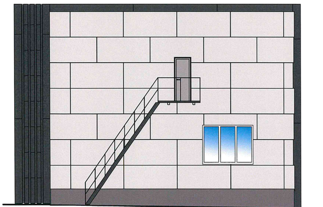
Боковой фасад
