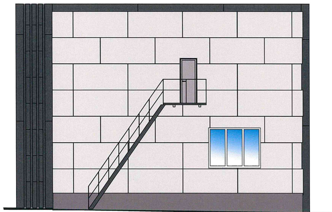
Боковой фасад
